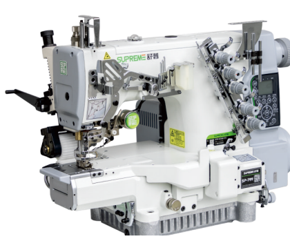
P PR P 后拉拖轮(齿状滚轮) Rear puller (toothed roller) PR 后拉拖轮(平状滚轮) Rear puller (flat roller)
